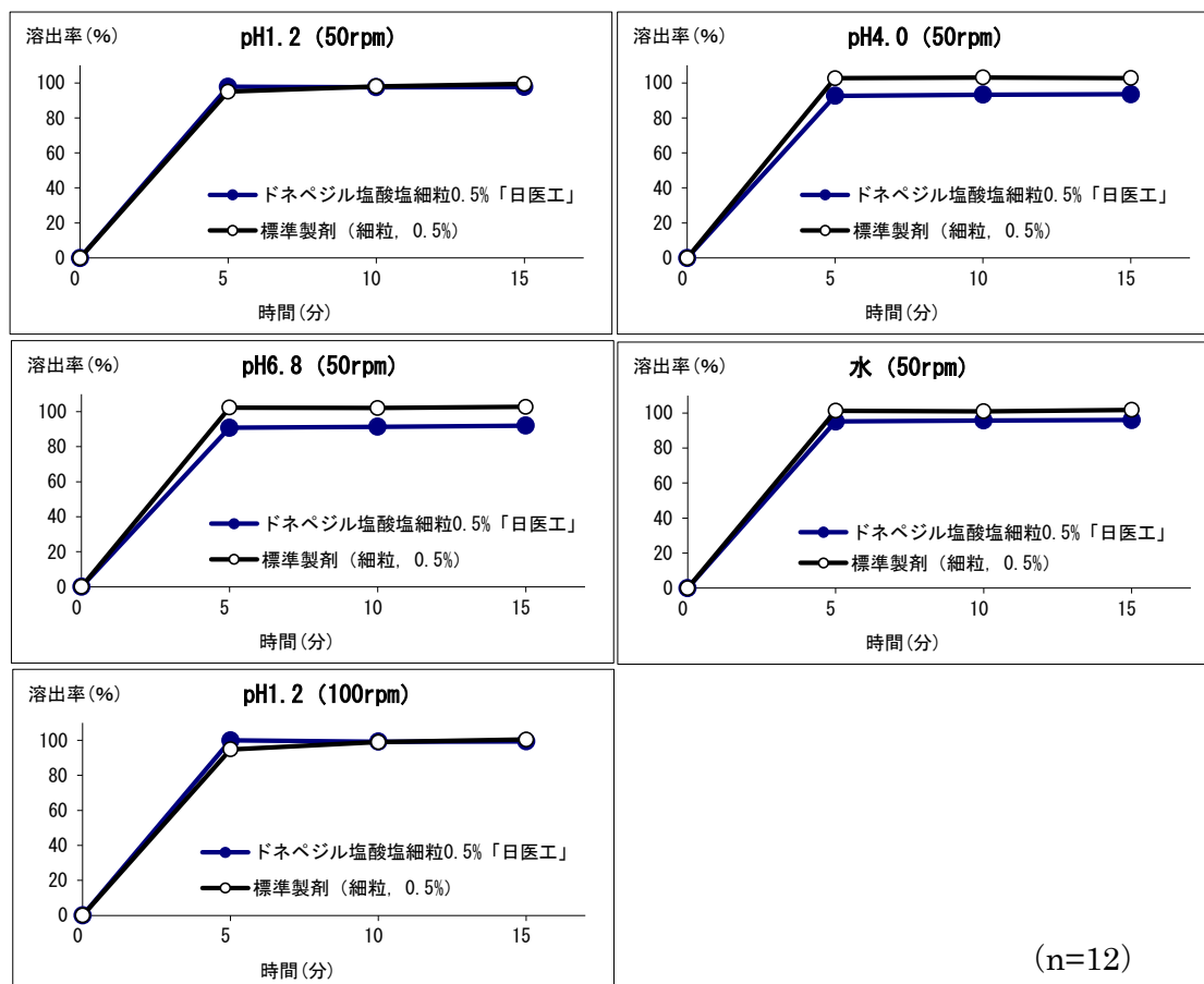
(溶出曲線)
