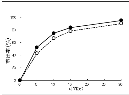
試験液 : pH4.0、50rpm
