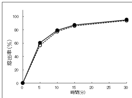
試験液 : pH4.0、100rpm
