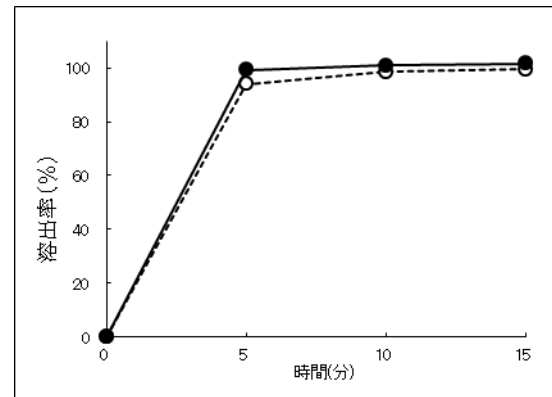
試験液 : pH6.8、50rpm
