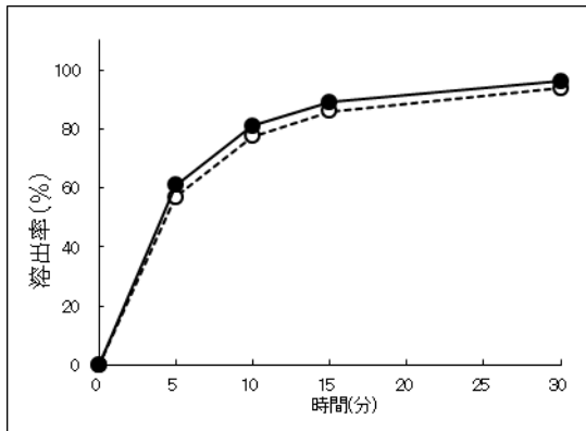
試験液：pH4.0、100rpm
