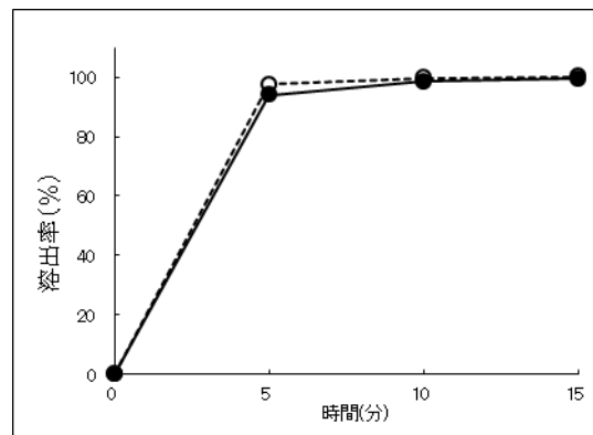
試験液:pH6.8、50rpm
