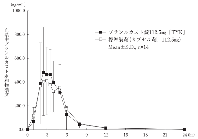
プランルカスト錠112.5mg「TYK」(2錠)投与後の血漿中濃度の推移
