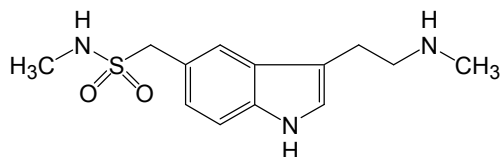
類縁物質 B の構造式
