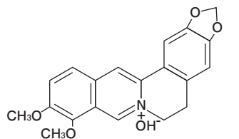
ベルベリン
