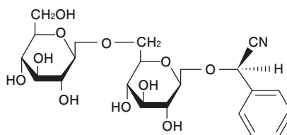
アミグダリン
