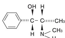
d -プソイドエフェドリン
