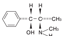
l -エフェドリン
