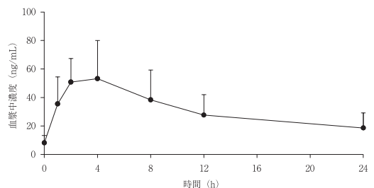
クロザピン25mg単回投与後の血漿中未変化体濃度推移
