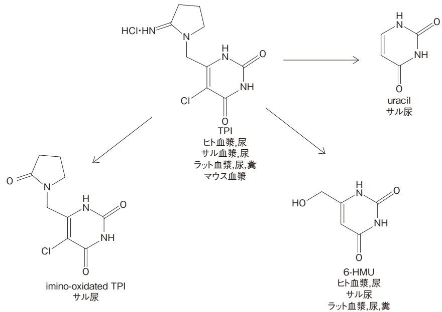
図VII-4 TPIの推定代謝経路
