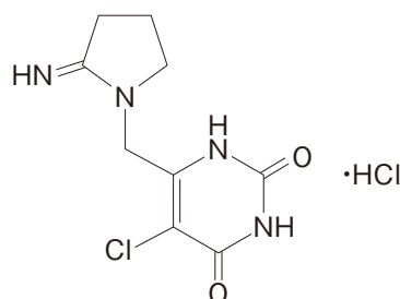
チピラシル塩酸塩
