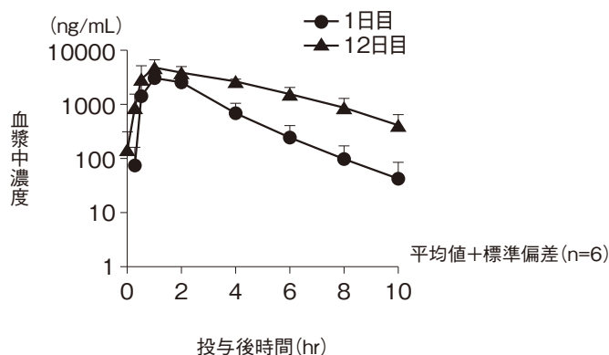
図VII-1 本剤を35mg/m 2 /回で単回投与及び1日2回反復投与したときの午前投与後の血漿中FTD濃度推移(J001試験)
