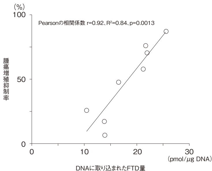
図VI-1 本剤の抗腫瘍効果とDNAに取り込まれたFTD量の相関関係
