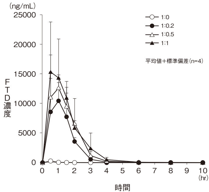
図VI-5 サルにFTD(10mg/kg)とTPIを各配合比で経口投与した後のFTDの血漿中濃度推移
