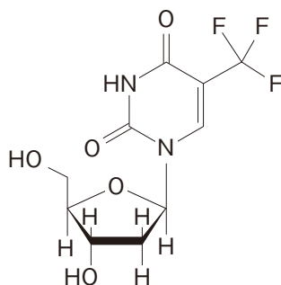
トリフルリジン
