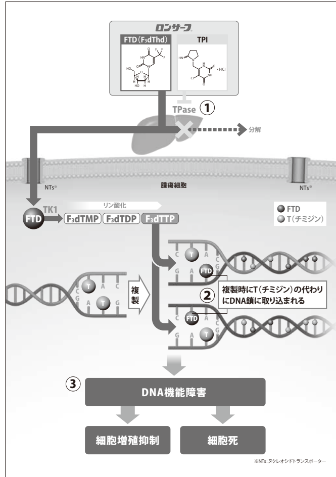
図Ⅵ-4 本剤の作用機序（イメージ図）（推定）
