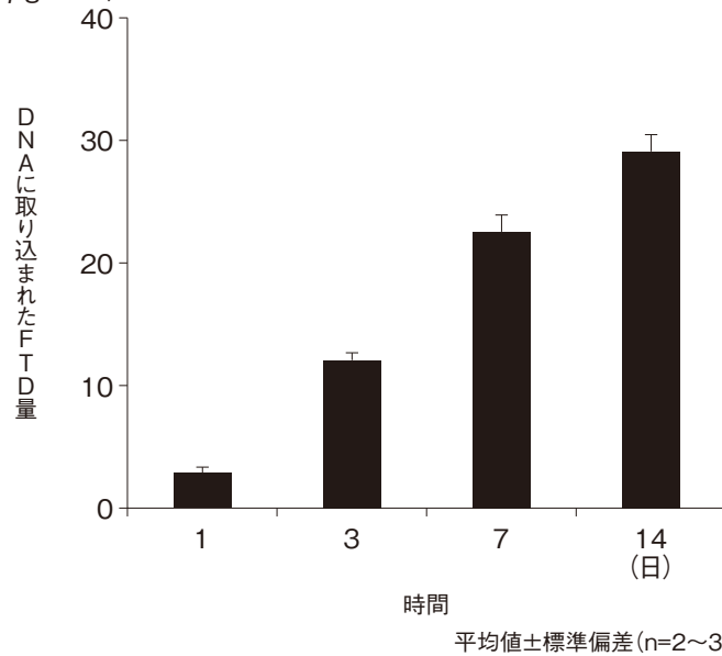
図VI-3 ヒト結腸・直腸癌由来KM20C細胞株のDNAに取り込まれたFTD量 (pmol/μg DNA)
