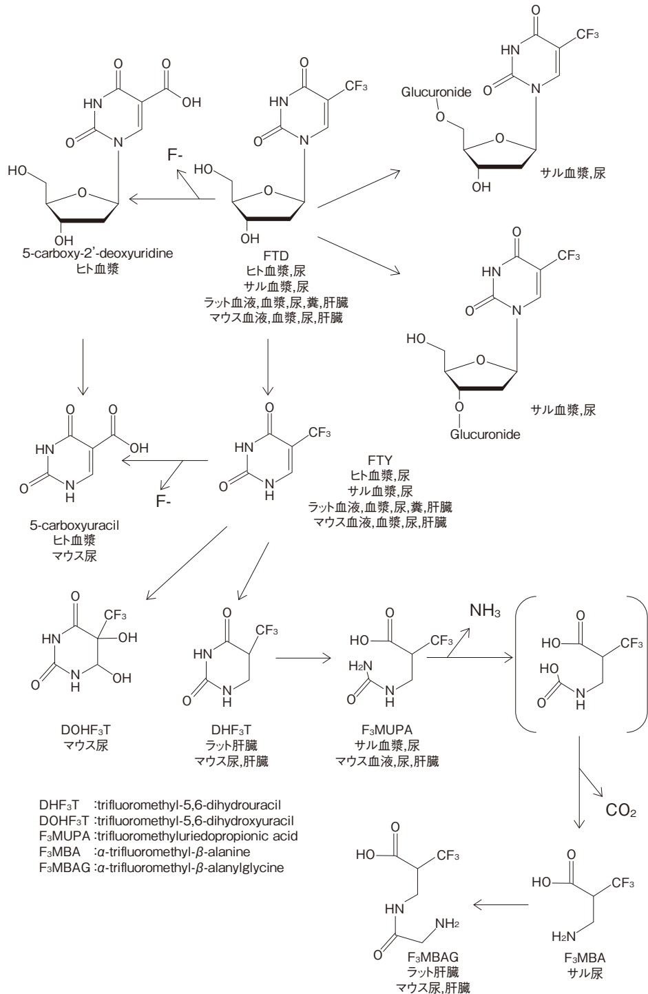
図VII-3 FTDの推定代謝経路
