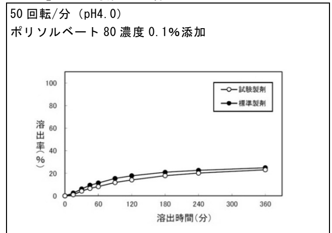
カンデサルタン錠 12mg 「サンド」 の平均溶出曲線
