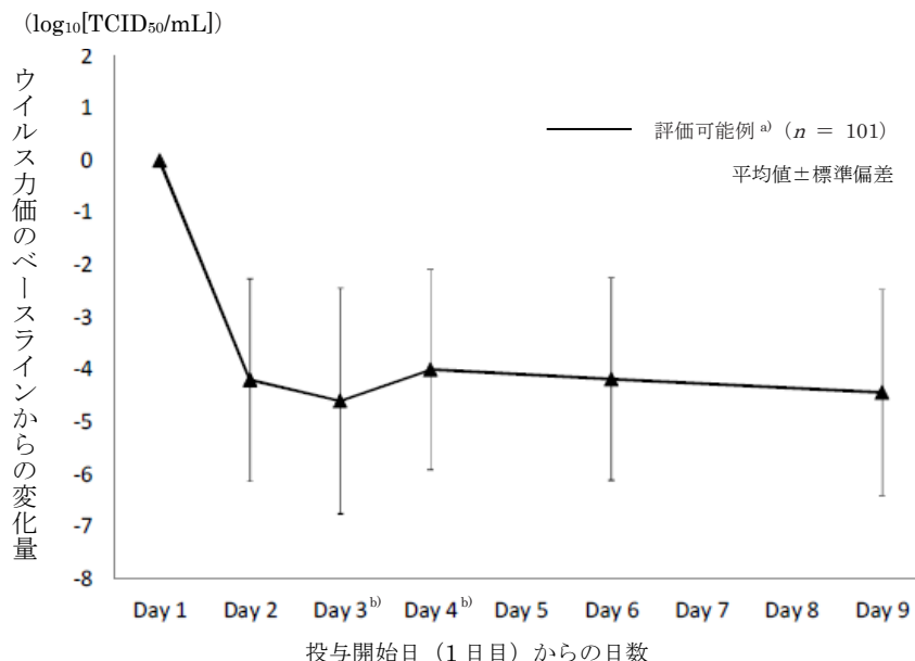
図V-11 ウイルス力価の変化量（ITTI）
