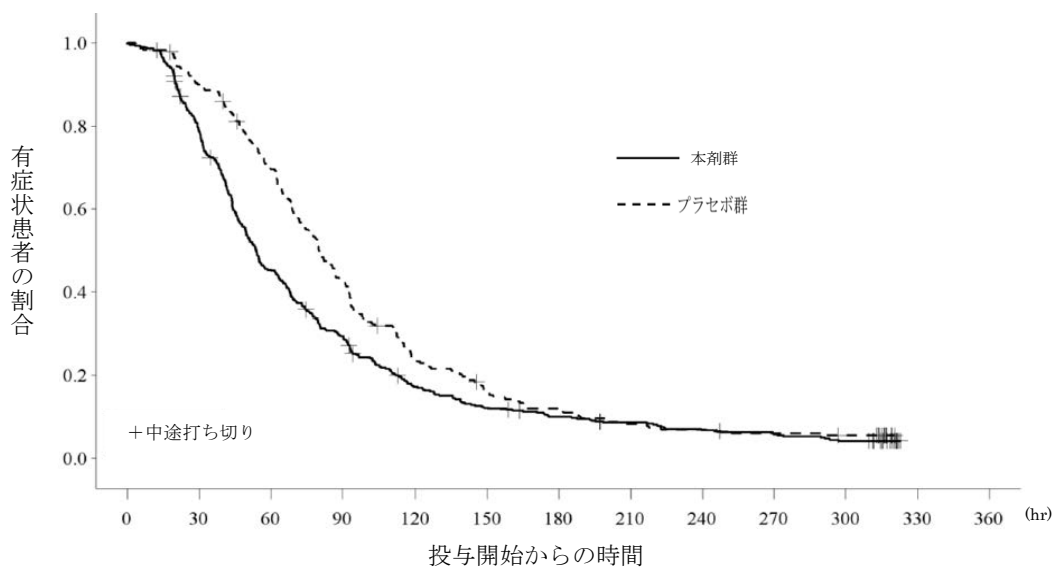
図V-4 12歳以上65歳未満患者におけるインフルエンザ罹病期間の Kaplan-Meier 曲線 (ITTI)
