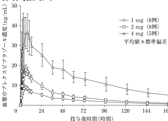
図16-1 健康成人におけるプレクスピプラゾール単回投与時の血漿中濃度推移
