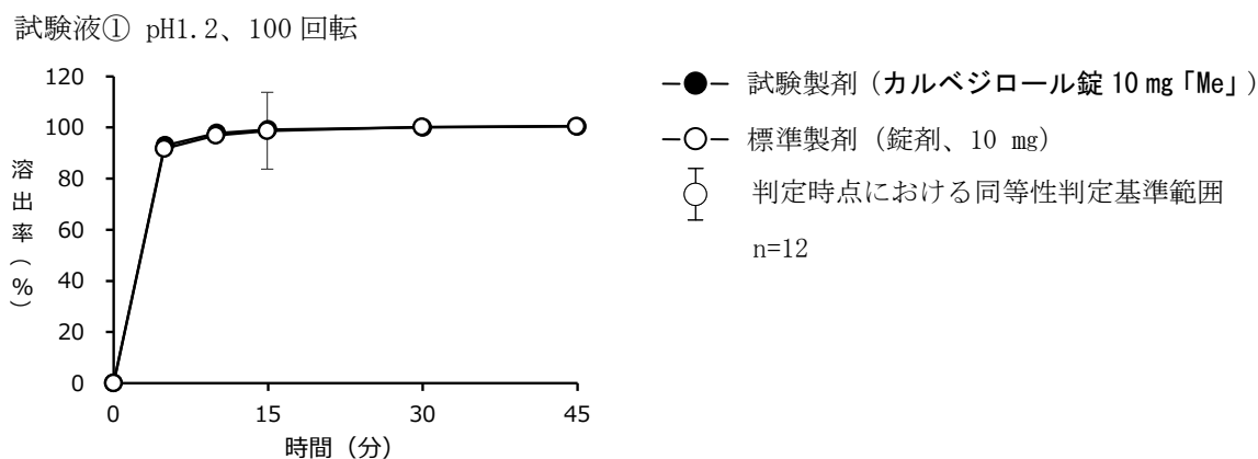
図 カルベジロール錠 10 mg 「Me」の溶出挙動における同等性 (試験製剤及び標準製剤の平均溶出率の比較)
