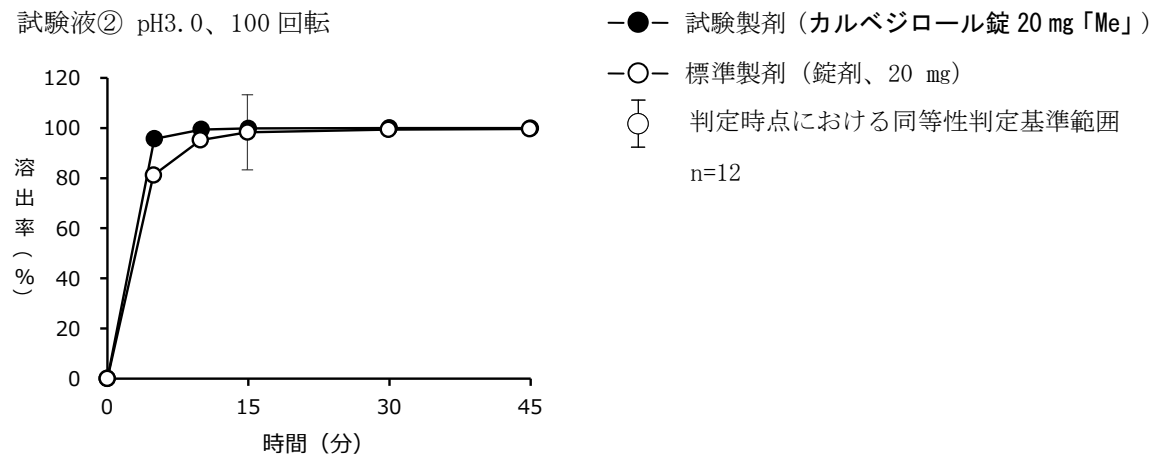
図 カルベジロール錠 20 mg 「Me」 の溶出挙動における同等性 (試験製剤及び標準製剤の平均溶出率の比較)
