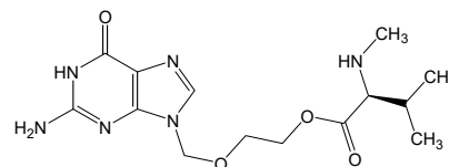
類縁物質 C(N-メチル体)
