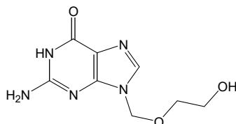
類縁物質 B(アシクロビル)
