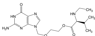
類縁物質 D(N-エチル体)
