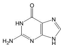
類縁物質 A(グアニン)
