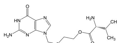
類縁物質 R(光学異性体)
