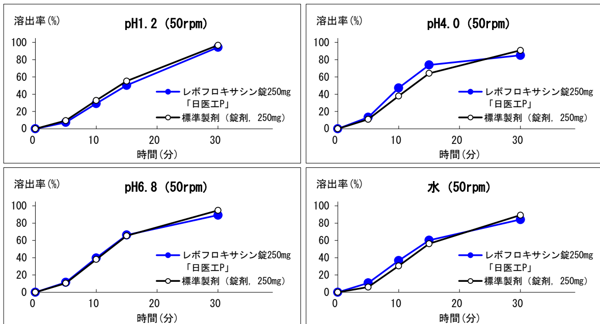
(溶出曲線)
