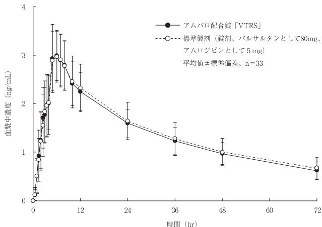
血漿中アムロジピン 濃度推移
