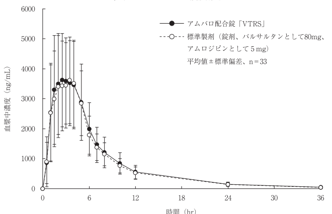
血漿中バルサルタン濃度推移
