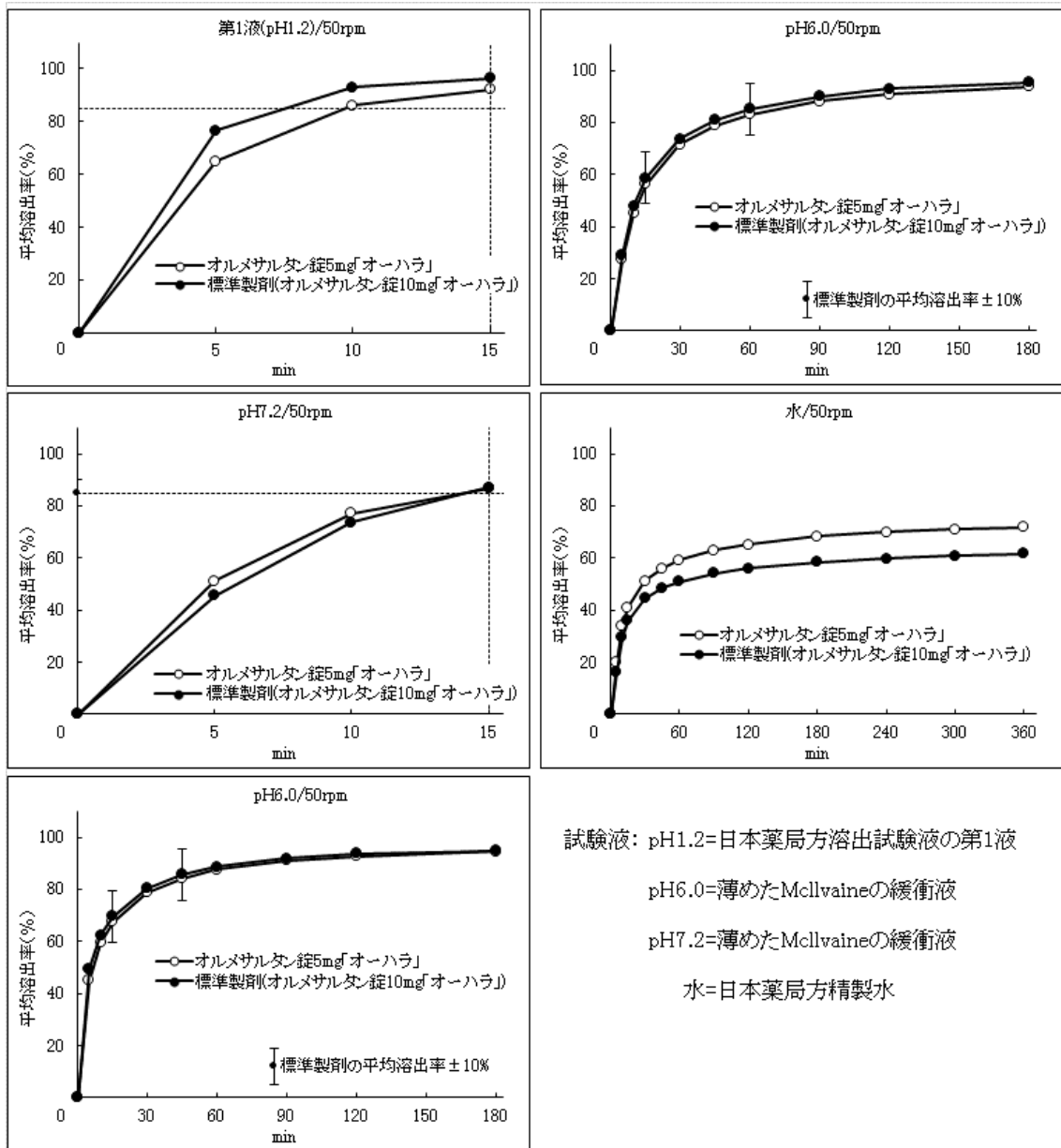
(溶出曲線)
