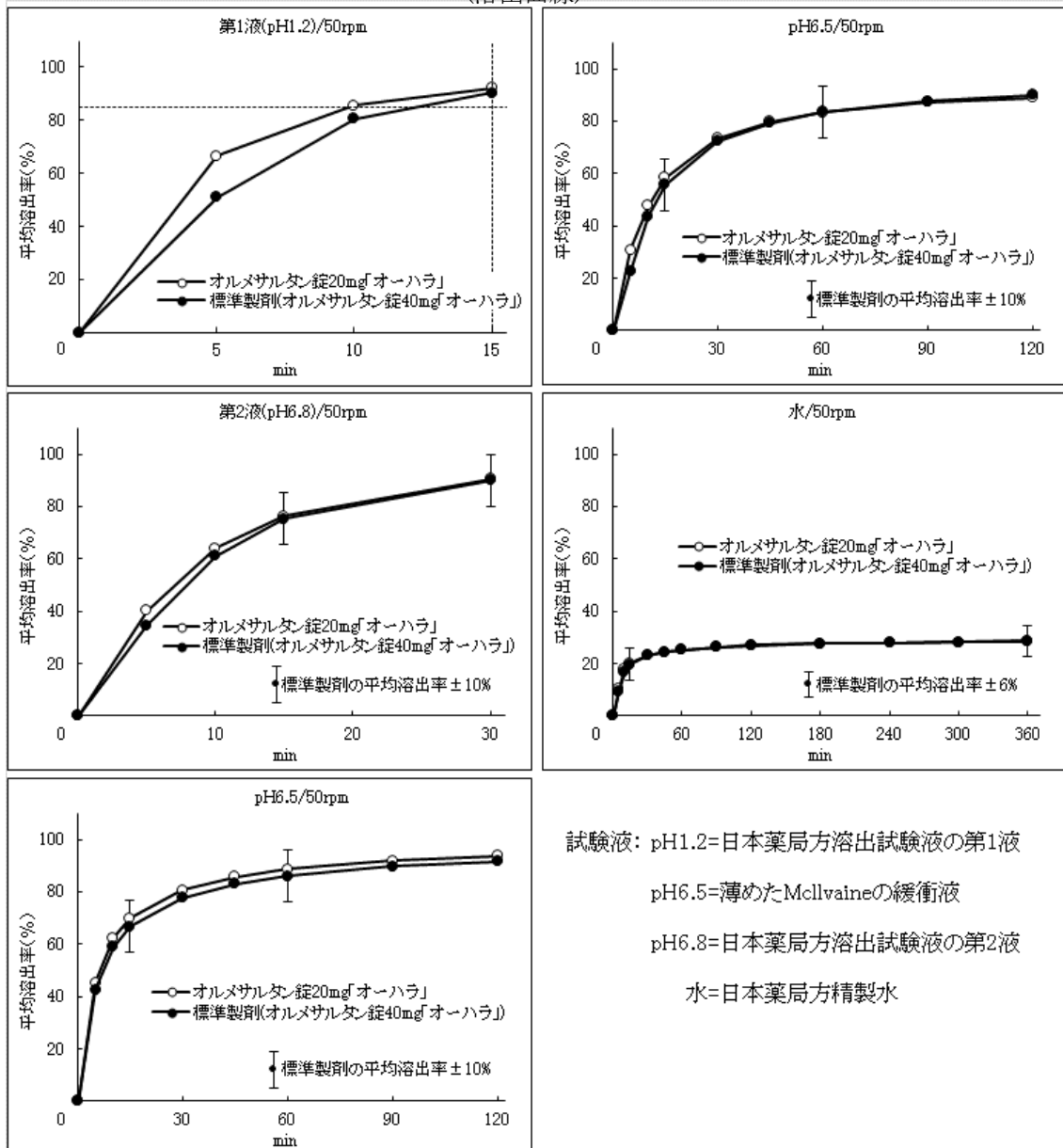
(溶出曲線)
