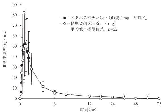
血漿中ビタバスタチンの濃度推移
