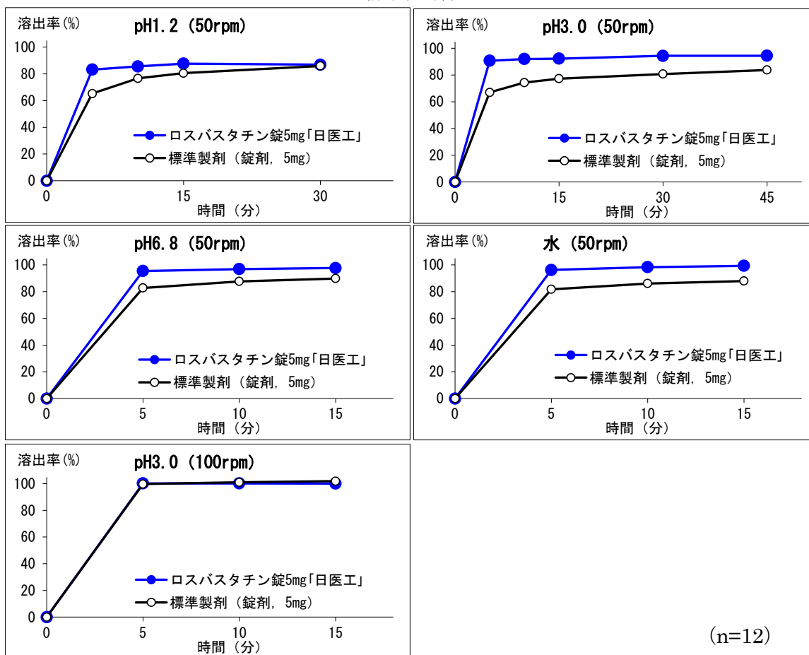
(溶出曲線)
