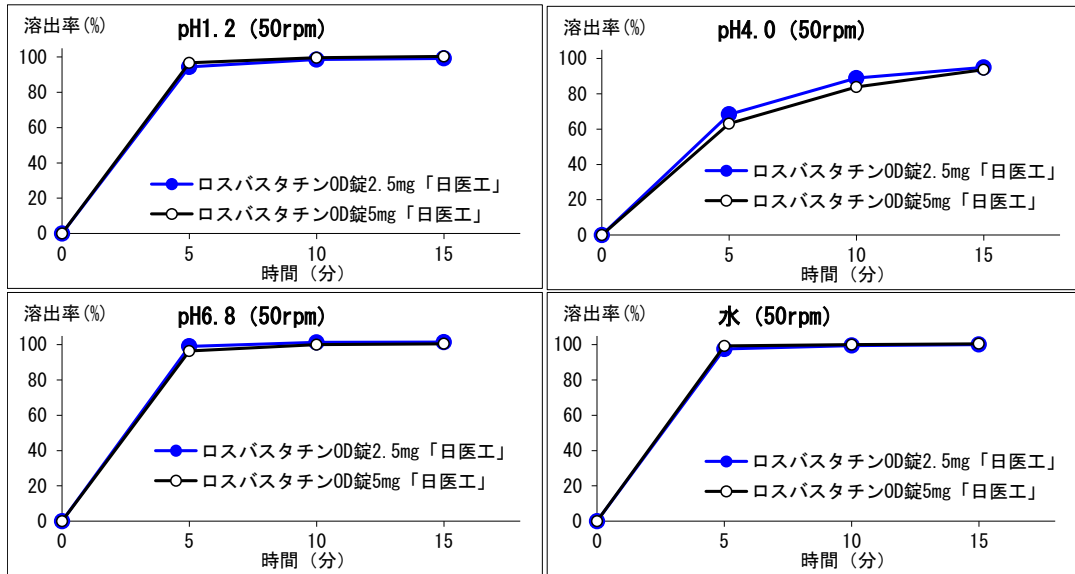
(溶出曲線)
