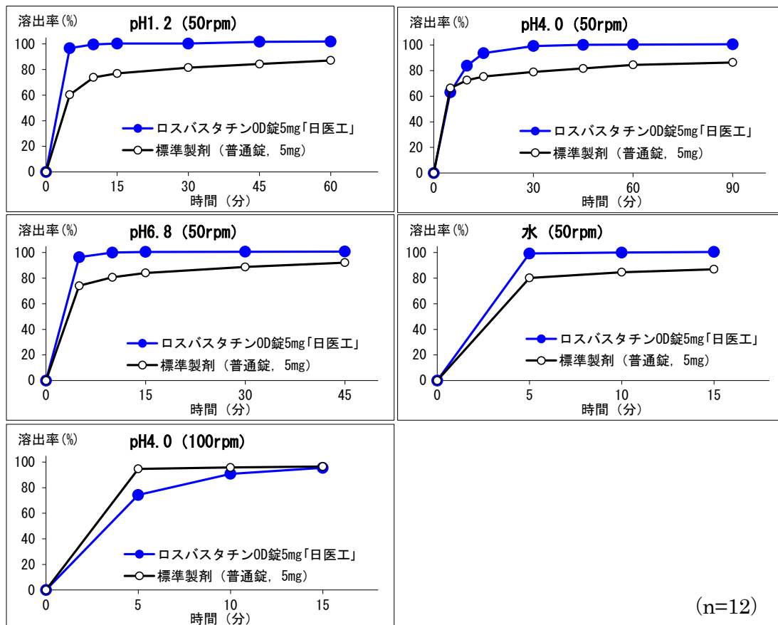
(溶出曲線)
