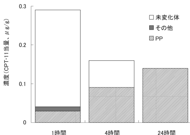
^{14}\text{C} -側鎖標識体（10mg/kg）静脈内投与後の未変化体とPPの脳内放射能濃度
