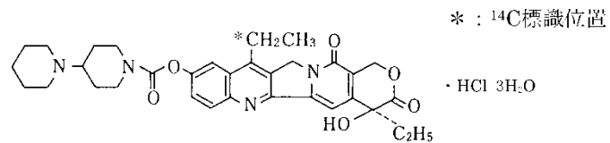
^{14}\text{C} -イリノテカン塩酸塩水和物 ( ^{14}\text{C} -標識体)
