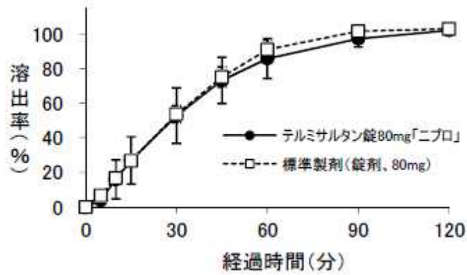
試験液 pH3.5 における平均溶出曲線 (mean \pm S. D.、n=12)
