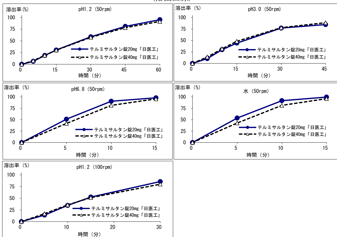
(溶出曲線)
