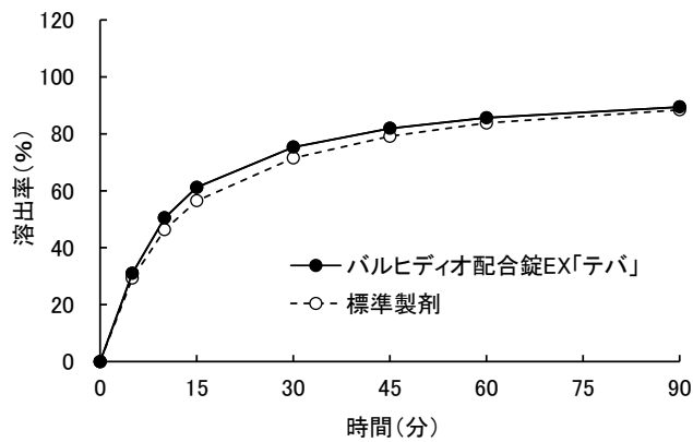
<pH3.0、100rpm>
