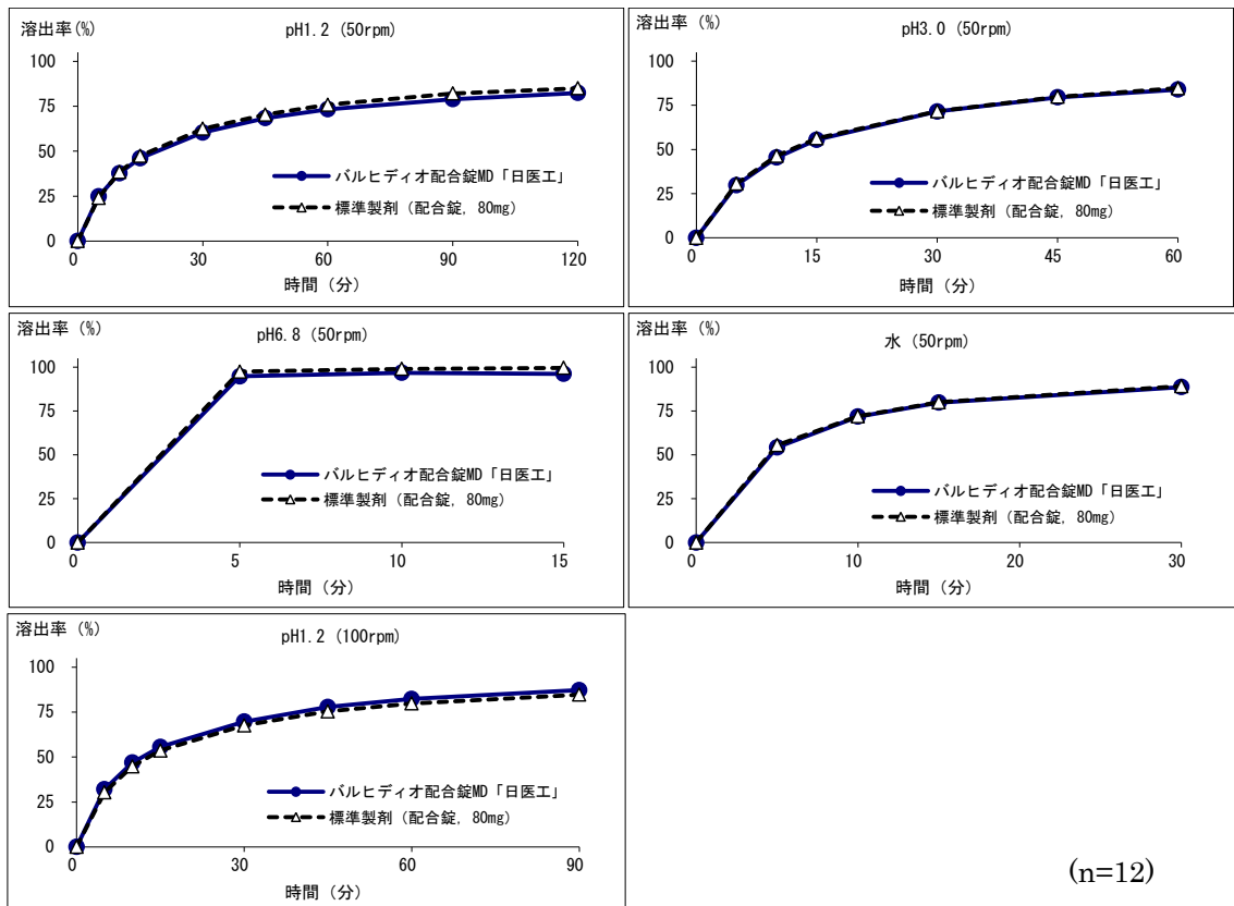
(溶出曲線)
