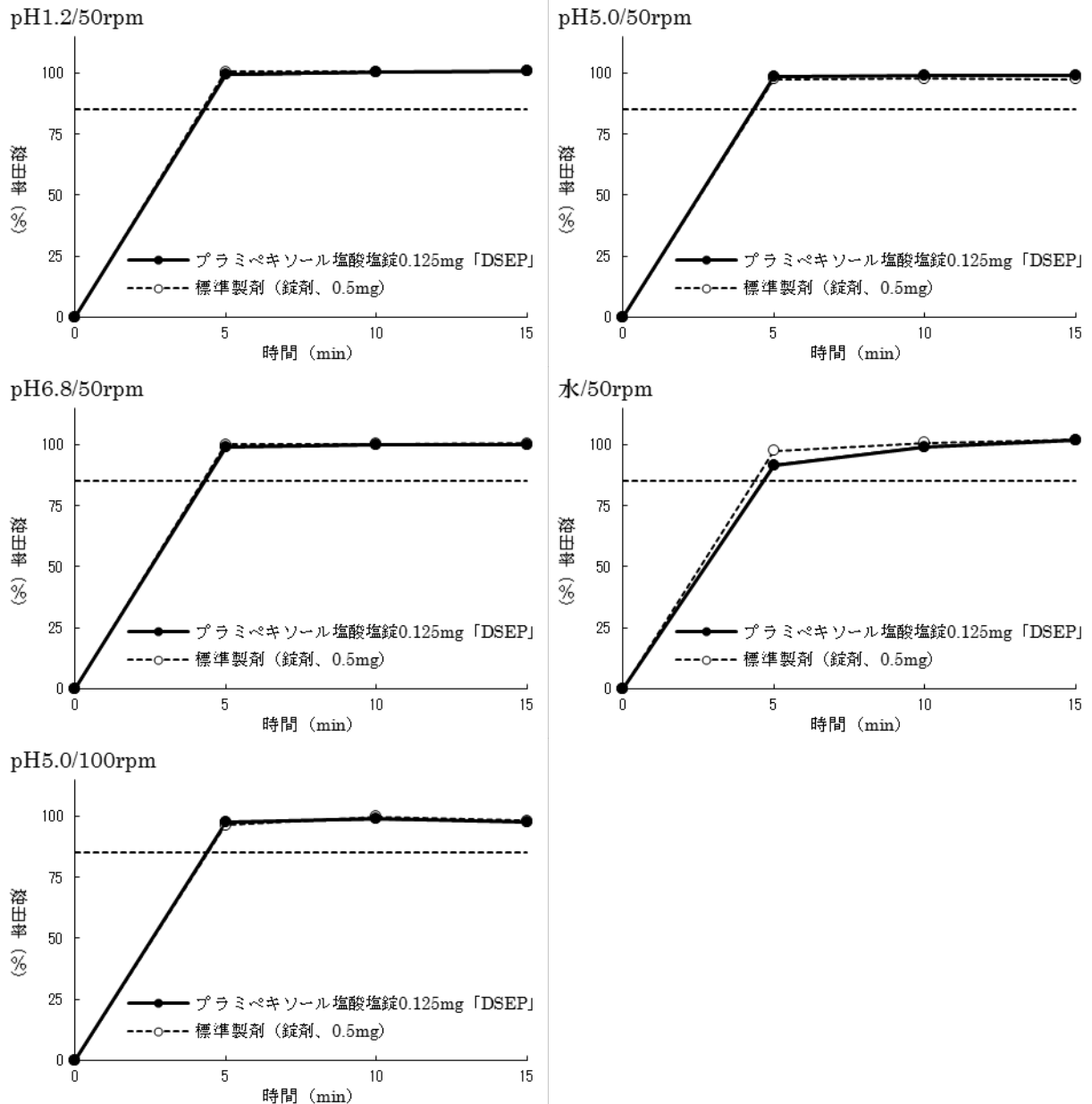
最終比較時点でのプラミペキソール塩酸塩錠 0.125mg 「DSEP」の個々の溶出率 (%)
