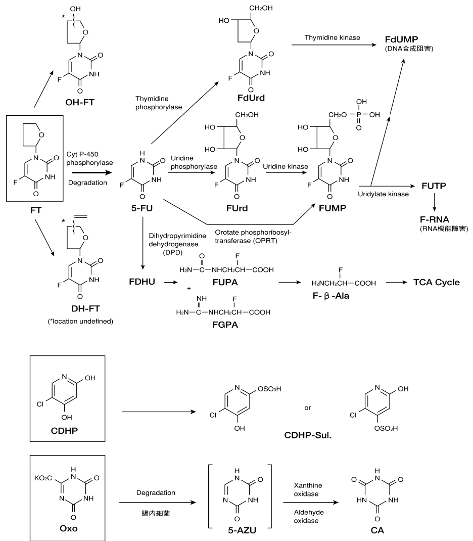
エスワントアイホウの配合成分 FT、CDHP、Oxo の推定代謝経路
