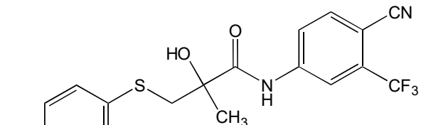
BICA III (合成中間体)
