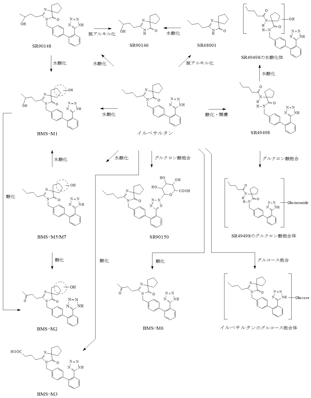
図VII-3 イレルベサルタンの推定代謝経路
