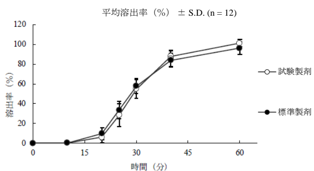
pH6.0*, 100rpm, パドル法
