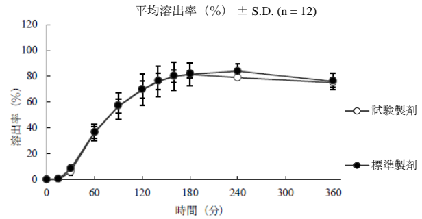
pH6.8*, 50rpm, パドル法
