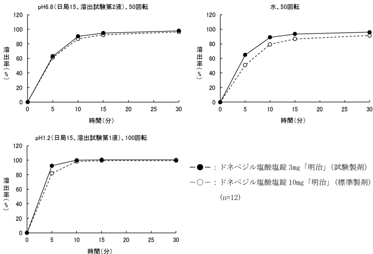
図IV-1 ドネペジル塩酸塩錠 3mg 「明治」 の溶出挙動における同等性 (試験製剤及び標準製剤の平均溶出率の比較)
