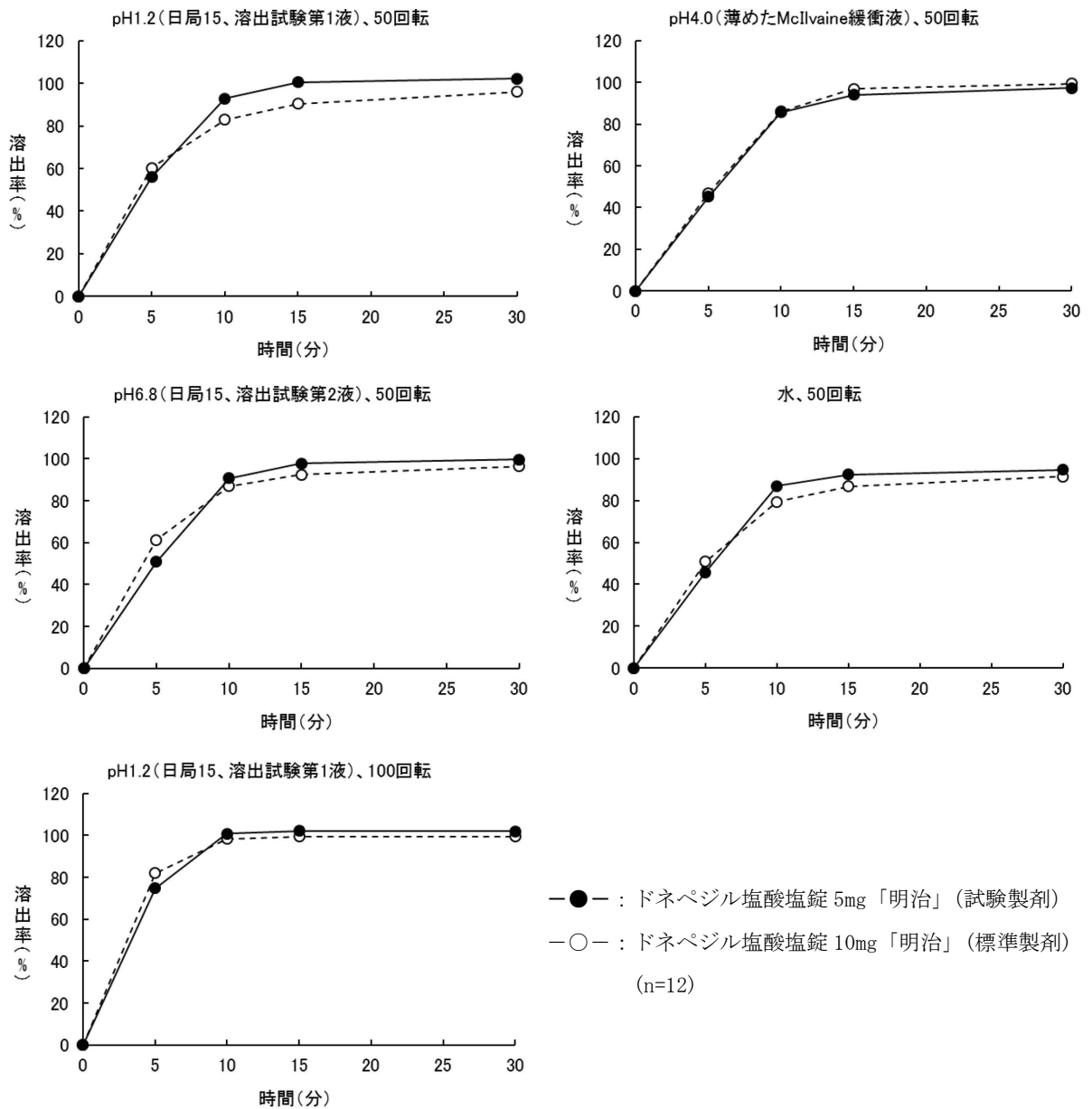
図Ⅳ-2 ドネペジル塩酸塩錠 5mg 「明治」の溶出挙動における同等性 (試験製剤及び標準製剤の平均溶出率の比較)
