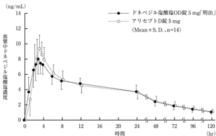
図VII-4 5mgOD錠投与時の血漿中ドネペジル塩酸塩濃度推移(水なし服用)
