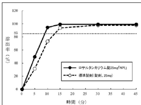
図5：pH5.0(100rpm)における溶出曲線
