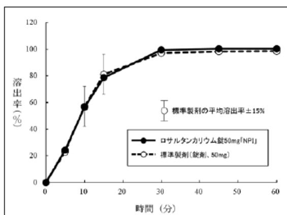
図3：pH6.8(50rpm)における溶出曲線
