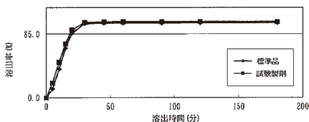
pH5.0 (100rpm) ロサルタンカリウム
