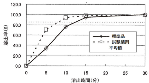
水 (50rpm)
