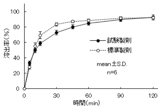
溶出試験結果 (1%SDS + pH6.8, 50rpm)
